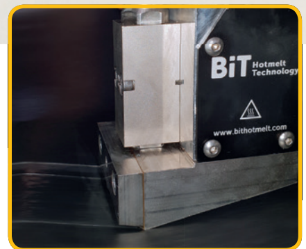
Lijmpatroon contact
